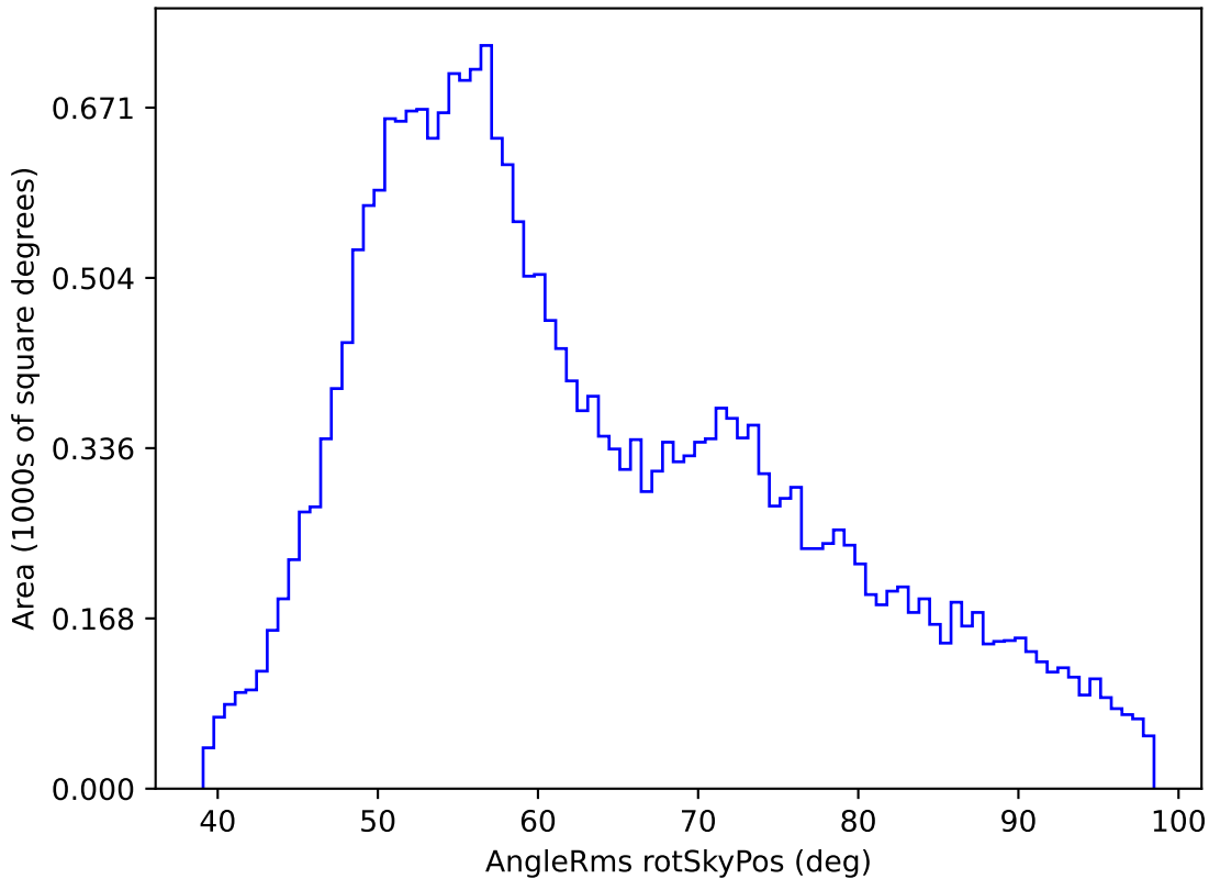
weather_cloudso36v3.4_10yrs All sky z band: AngleRms rotSkyPos
