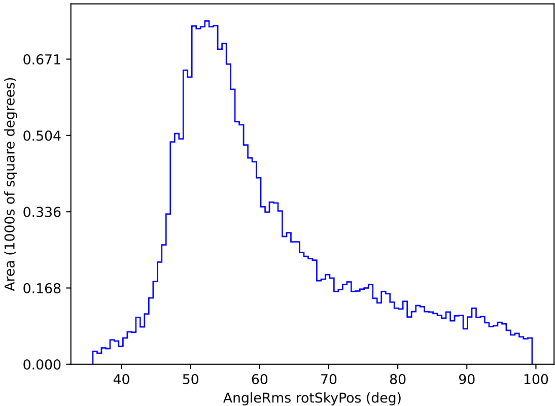
weather_cloudso36v3.4_10yrs All sky y band: AngleRms rotSkyPos
