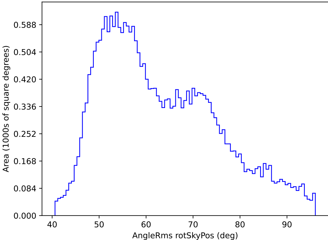
weather_cloudso36v3.4_10yrs All sky i band: AngleRms rotSkyPos
