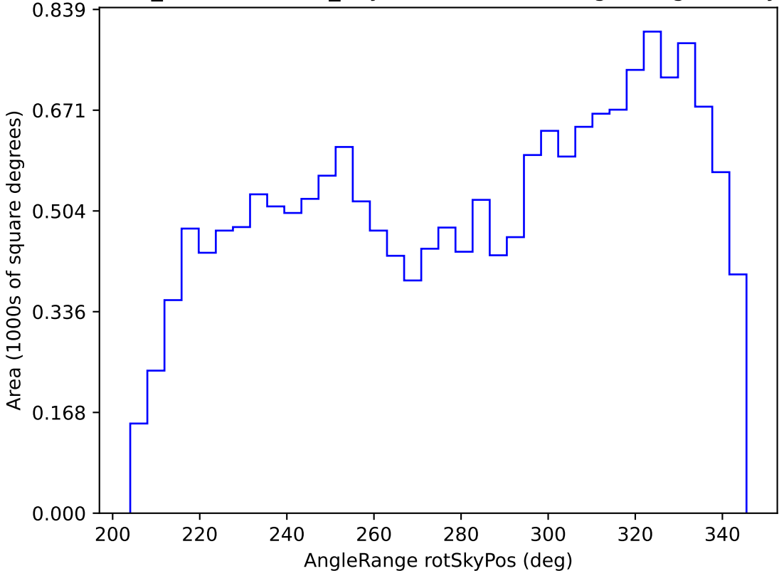
weather_cloudso36v3.4_10yrs WFD z band: AngleRange rotSkyPos
