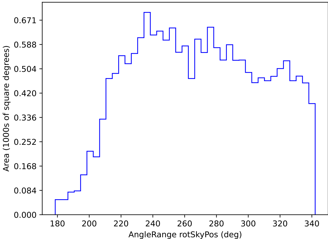
weather_cloudso36v3.4_10yrs WFD y band: AngleRange rotSkyPos
