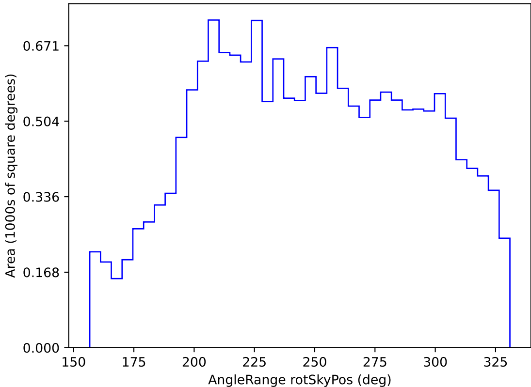
weather_cloudso36v3.4_10yrs WFD u band: AngleRange rotSkyPos
