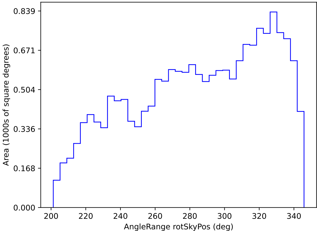
weather_cloudso36v3.4_10yrs WFD r band: AngleRange rotSkyPos
