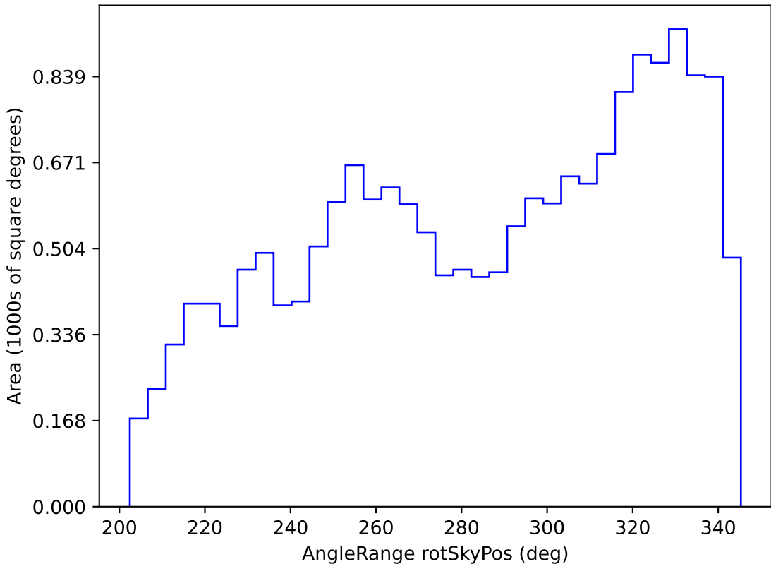
weather_cloudso36v3.4_10yrs WFD i band: AngleRange rotSkyPos
