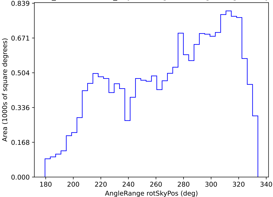
weather_cloudso36v3.4_10yrs WFD g band: AngleRange rotSkyPos
