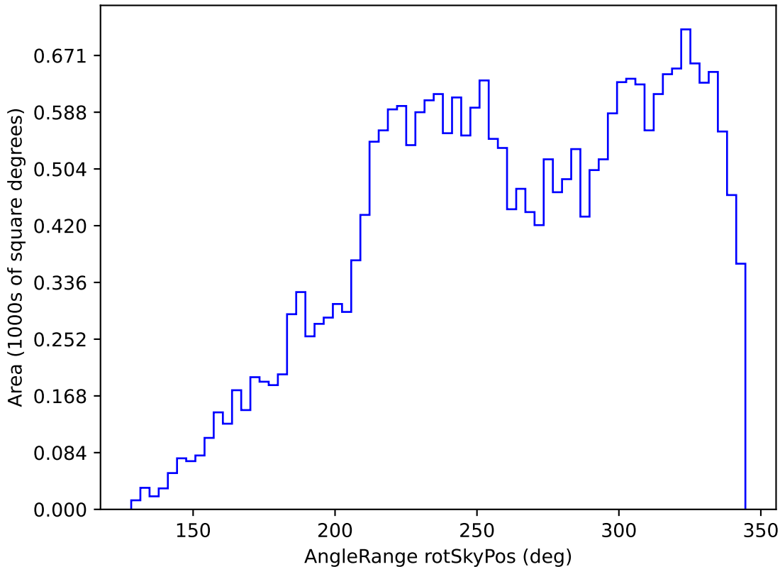
weather_cloudso36v3.4_10yrs All sky z band: AngleRange rotSkyPos
