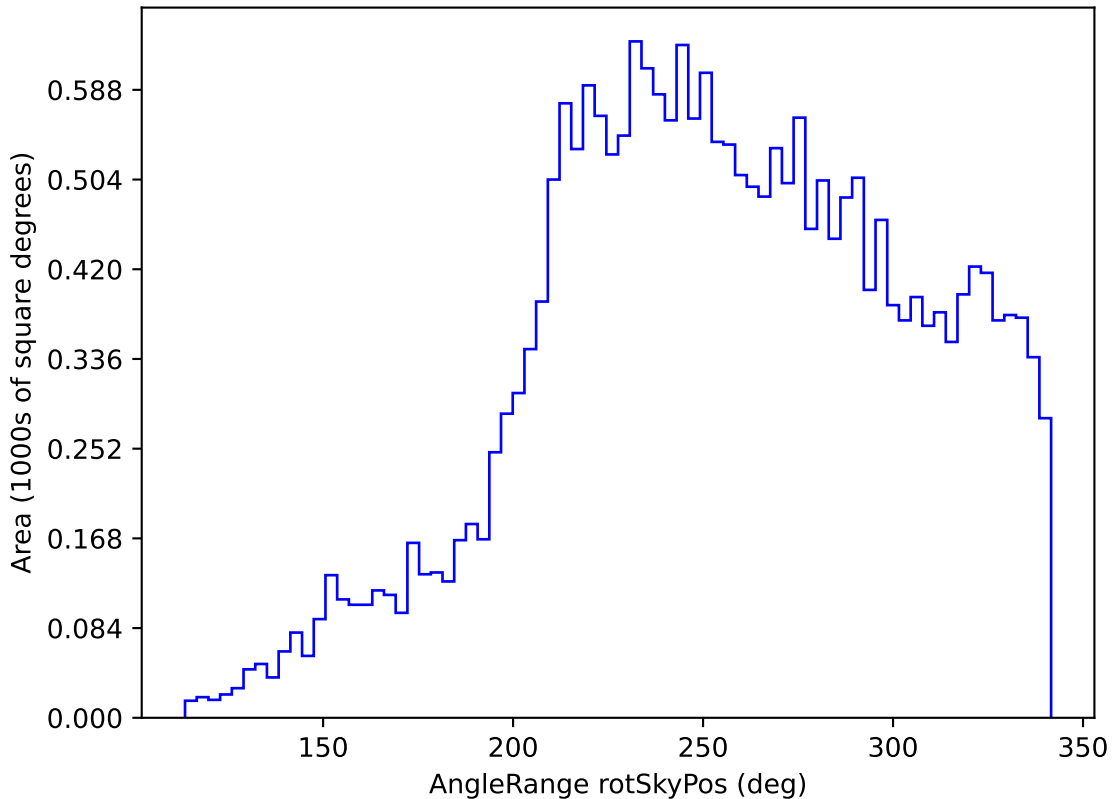
weather_cloudso36v3.4_10yrs All sky y band: AngleRange rotSkyPos
