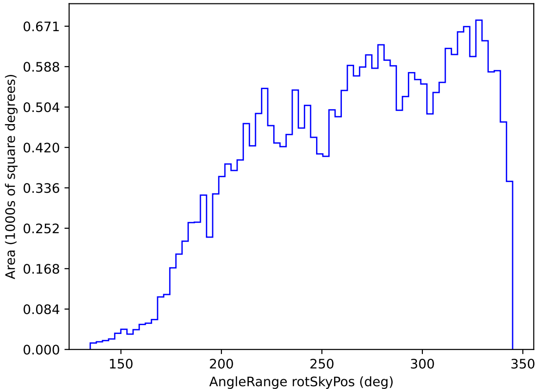
weather_cloudso36v3.4_10yrs All sky r band: AngleRange rotSkyPos
