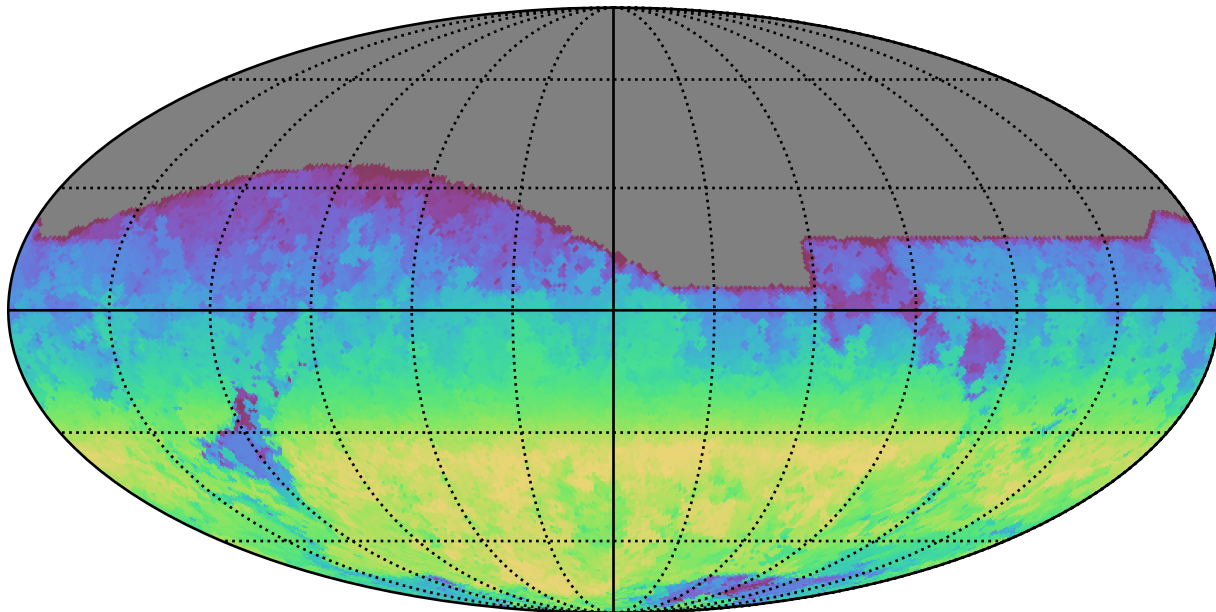
weather_cloudso36v3.4_10yrs All sky i band: AngleRange rotSkyPos
