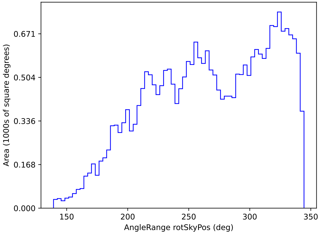
weather_cloudso36v3.4_10yrs All sky i band: AngleRange rotSkyPos
