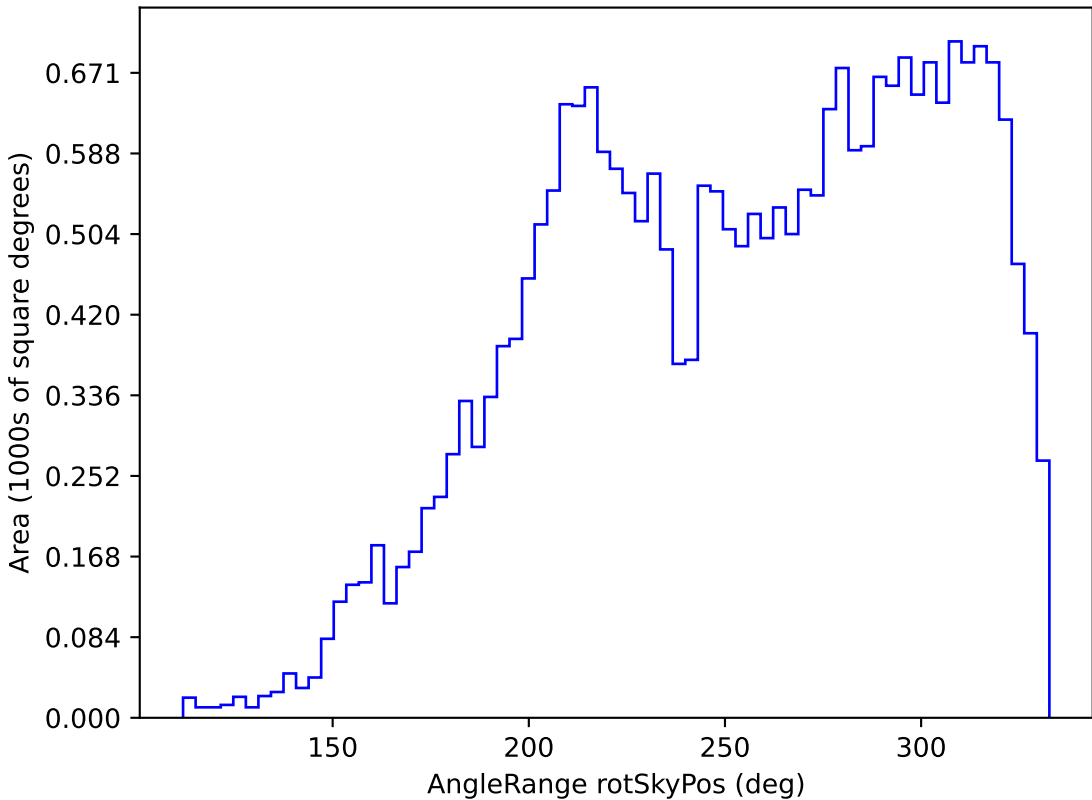
weather_cloudso36v3.4_10yrs All sky g band: AngleRange rotSkyPos
