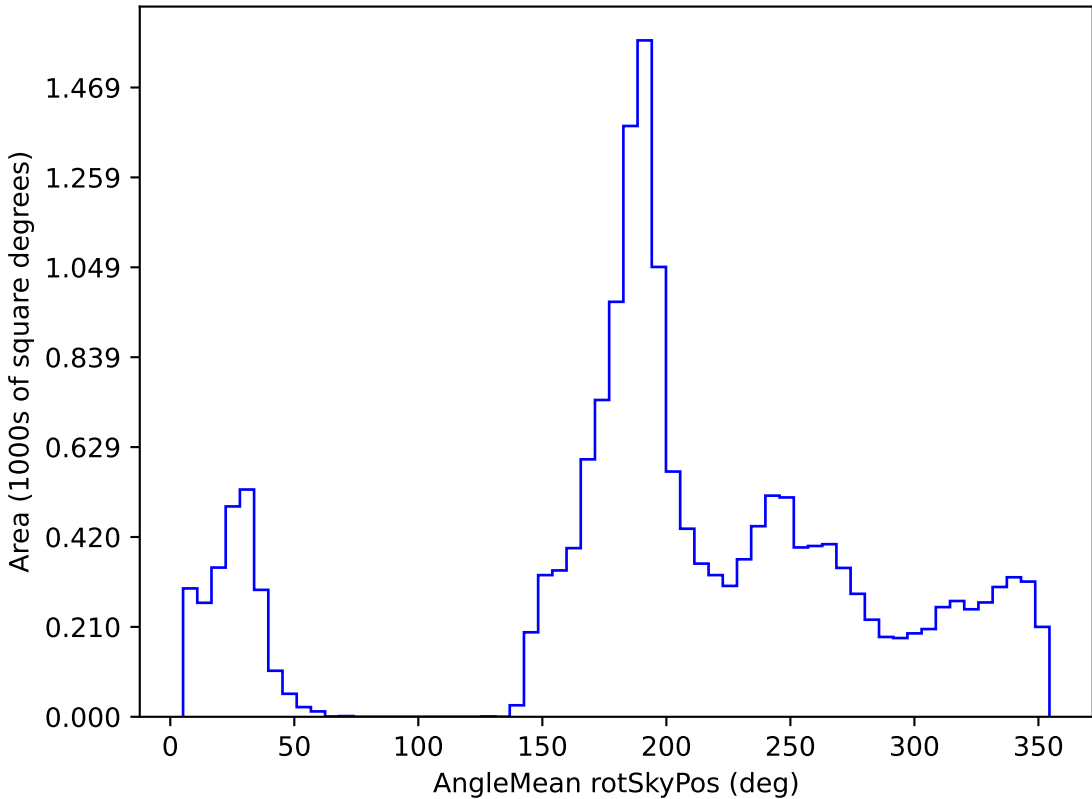
weather_cloudso36v3.4_10yrs WFD z band: AngleMean rotSkyPos
