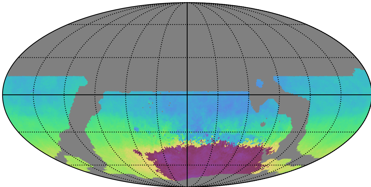
weather_cloudso36v3.4_10yrs WFD y band: AngleMean rotSkyPos
