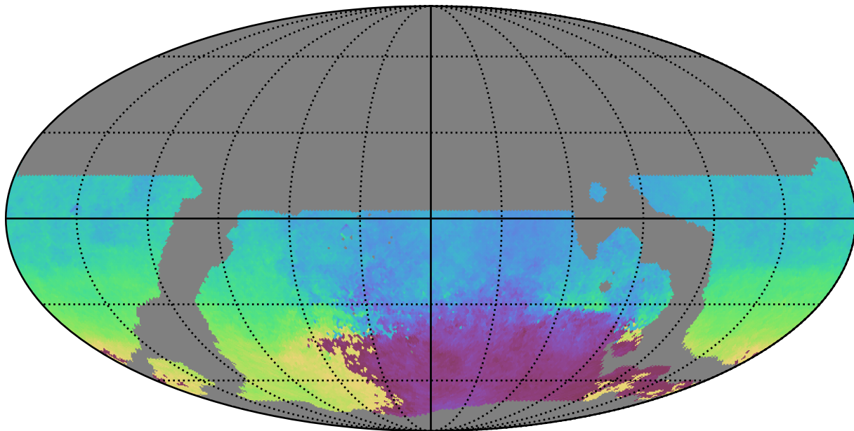
weather_cloudso36v3.4_10yrs WFD u band: AngleMean rotSkyPos
