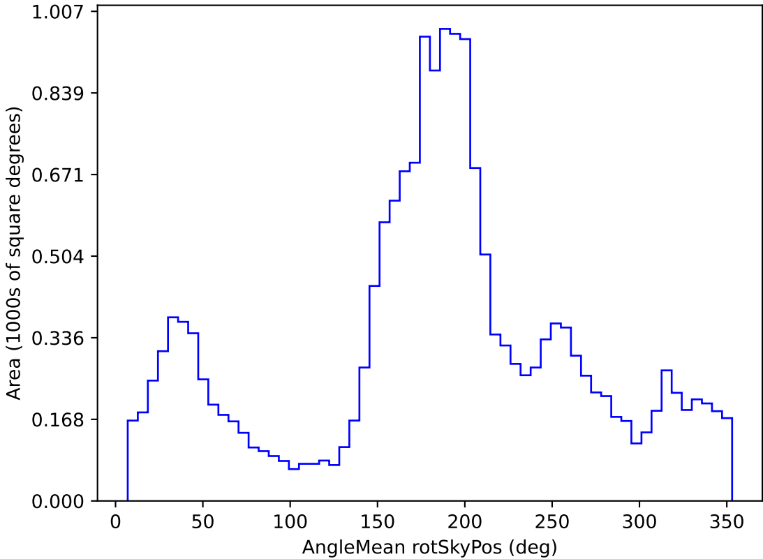
weather_cloudso36v3.4_10yrs WFD u band: AngleMean rotSkyPos
