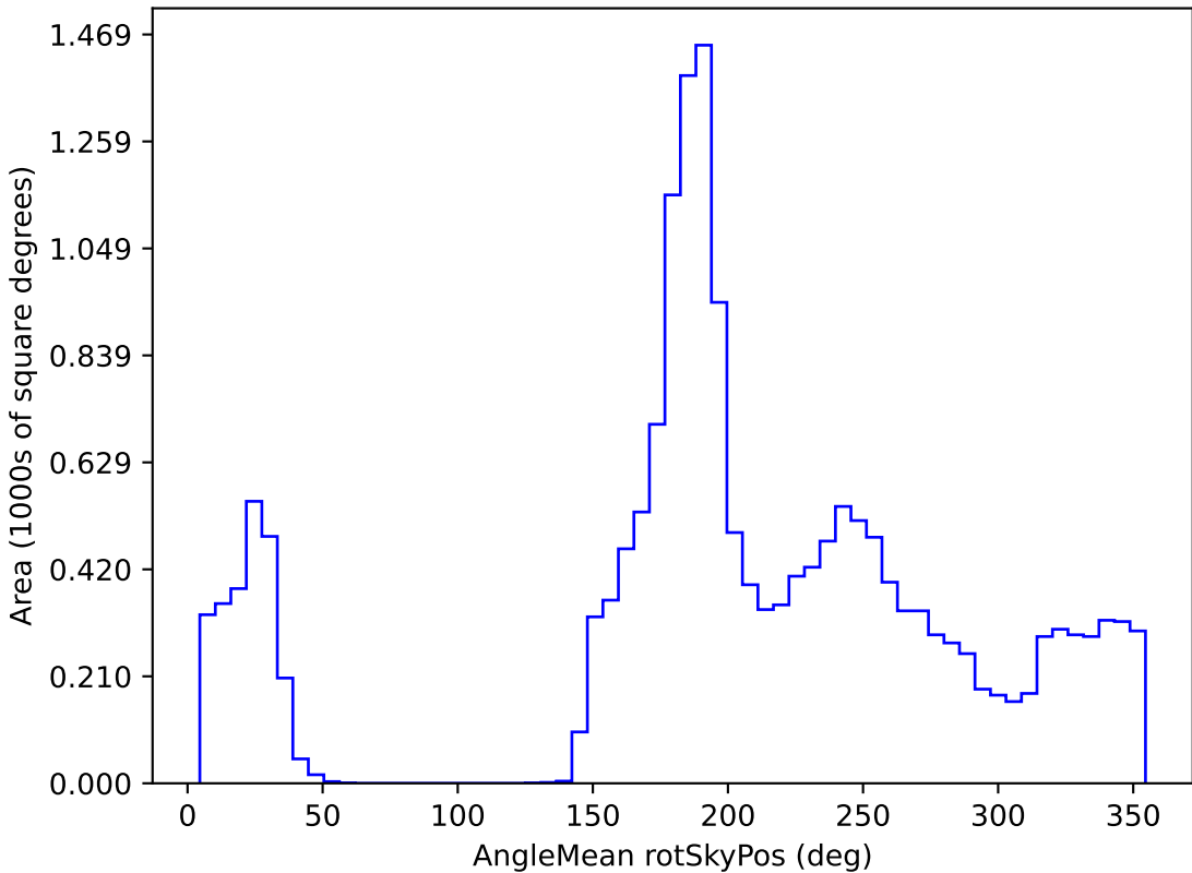
weather_cloudso36v3.4_10yrs WFD i band: AngleMean rotSkyPos
