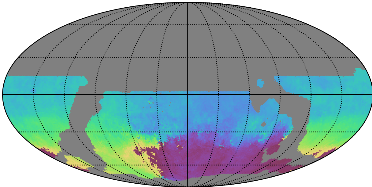
weather_cloudso36v3.4_10yrs WFD g band: AngleMean rotSkyPos
