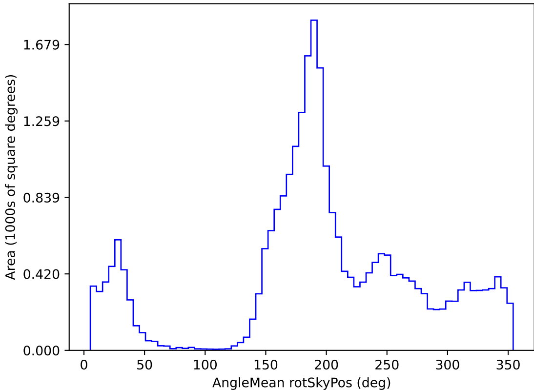
weather_cloudso36v3.4_10yrs All sky z band: AngleMean rotSkyPos
