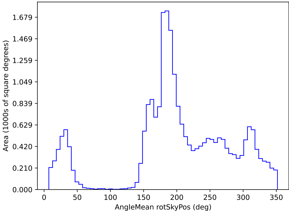
weather_cloudso36v3.4_10yrs All sky y band: AngleMean rotSkyPos
