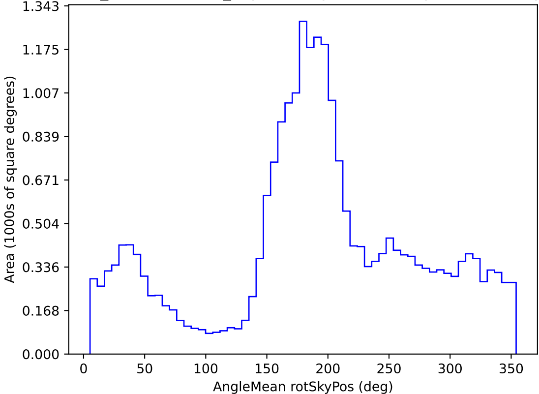
weather_cloudso36v3.4_10yrs All sky u band: AngleMean rotSkyPos
