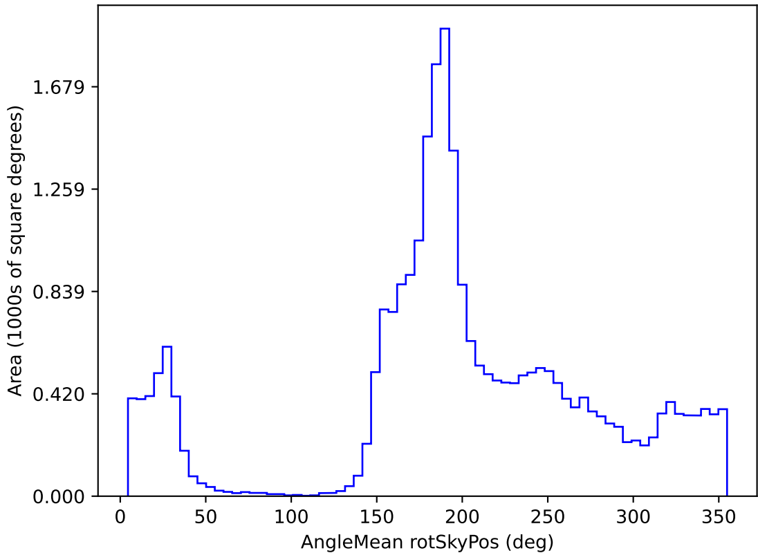
weather_cloudso36v3.4_10yrs All sky i band: AngleMean rotSkyPos
