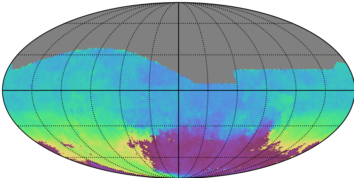
weather_cloudso36v3.4_10yrs All sky g band: AngleMean rotSkyPos
