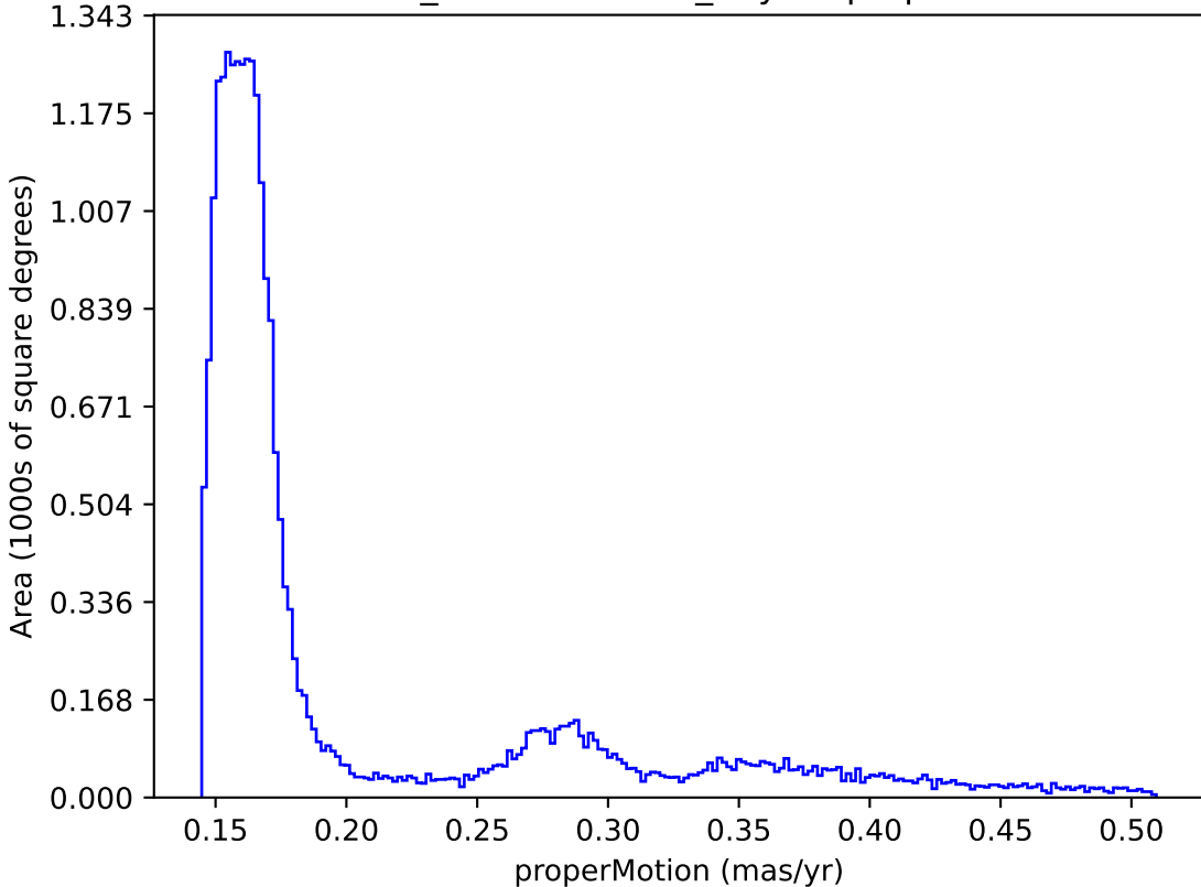
weather_cloudso36v3.4_10yrs : properMotion
