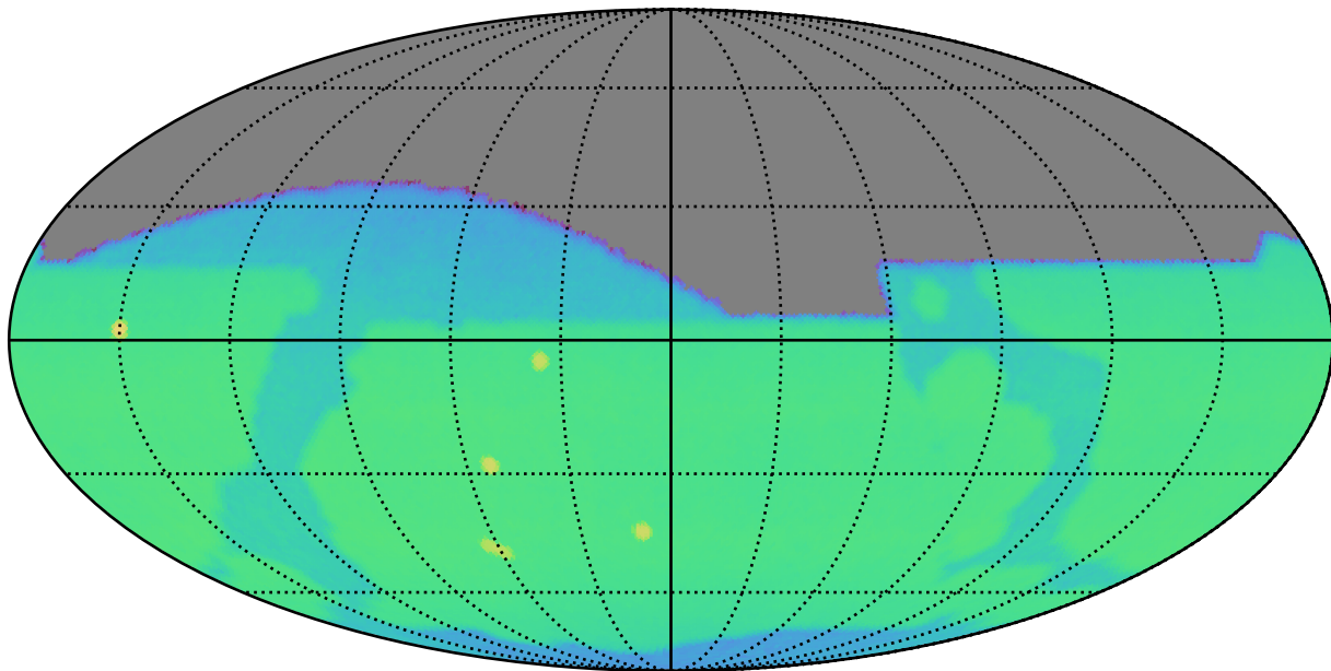
weather_cloudso36v3.4_10yrs i: CoaddM5
