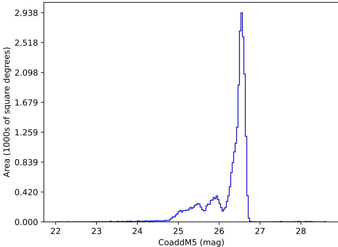
weather_cloudso36v3.4_10yrs i: CoaddM5
