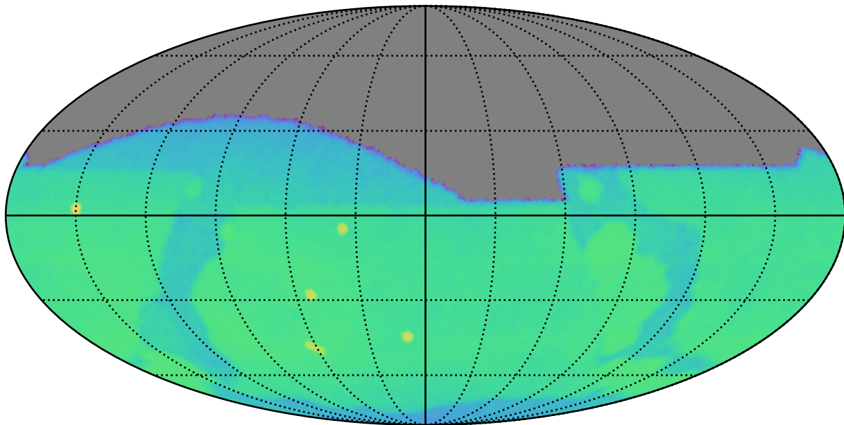
weather_cloudso36v3.4_10yrs g: CoaddM5
