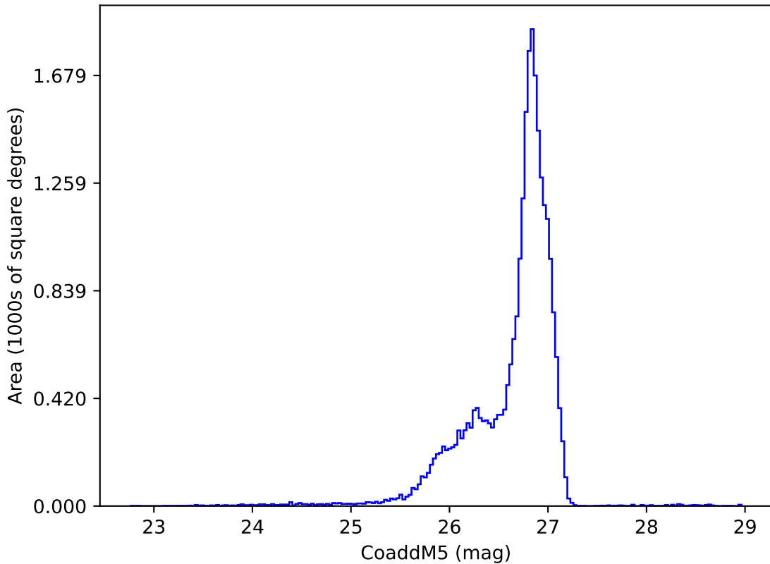
weather_cloudso36v3.4_10yrs g: CoaddM5
