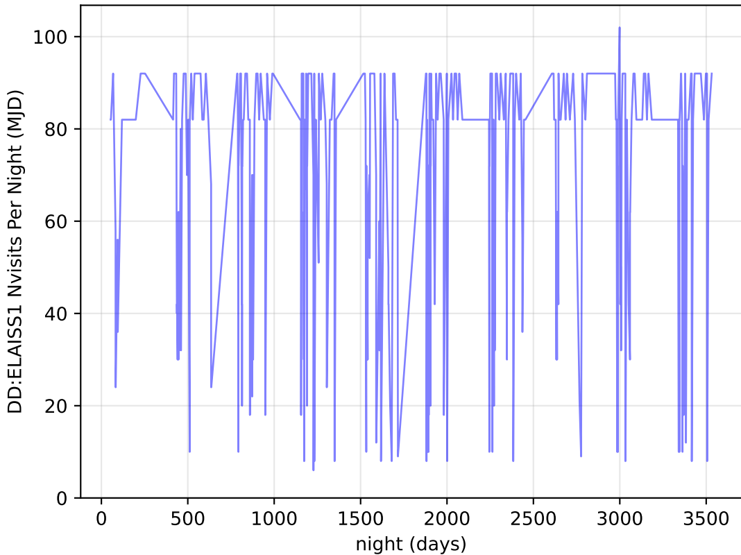
weather_cloudso36v3.4_10yrs all bands: DD:ELAISS1 Nvisits Per Night
