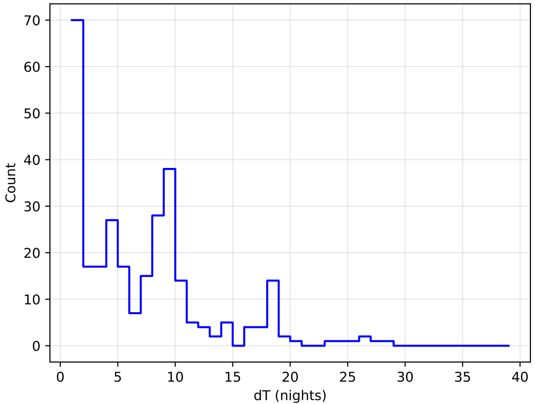
weather_cloudso36v3.4_10yrs all bands: DD:ELAISS1 Delta Nights Histogram
