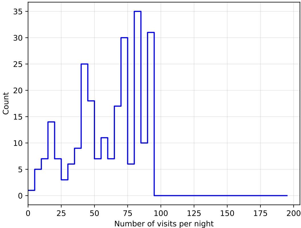
weather_cloudso36v3.4_10yrs all bands: DD:EDFS NVisitsPerNight
