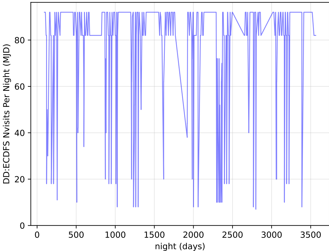
weather_cloudso36v3.4_10yrs all bands: DD:ECDFS Nvisits Per Night
