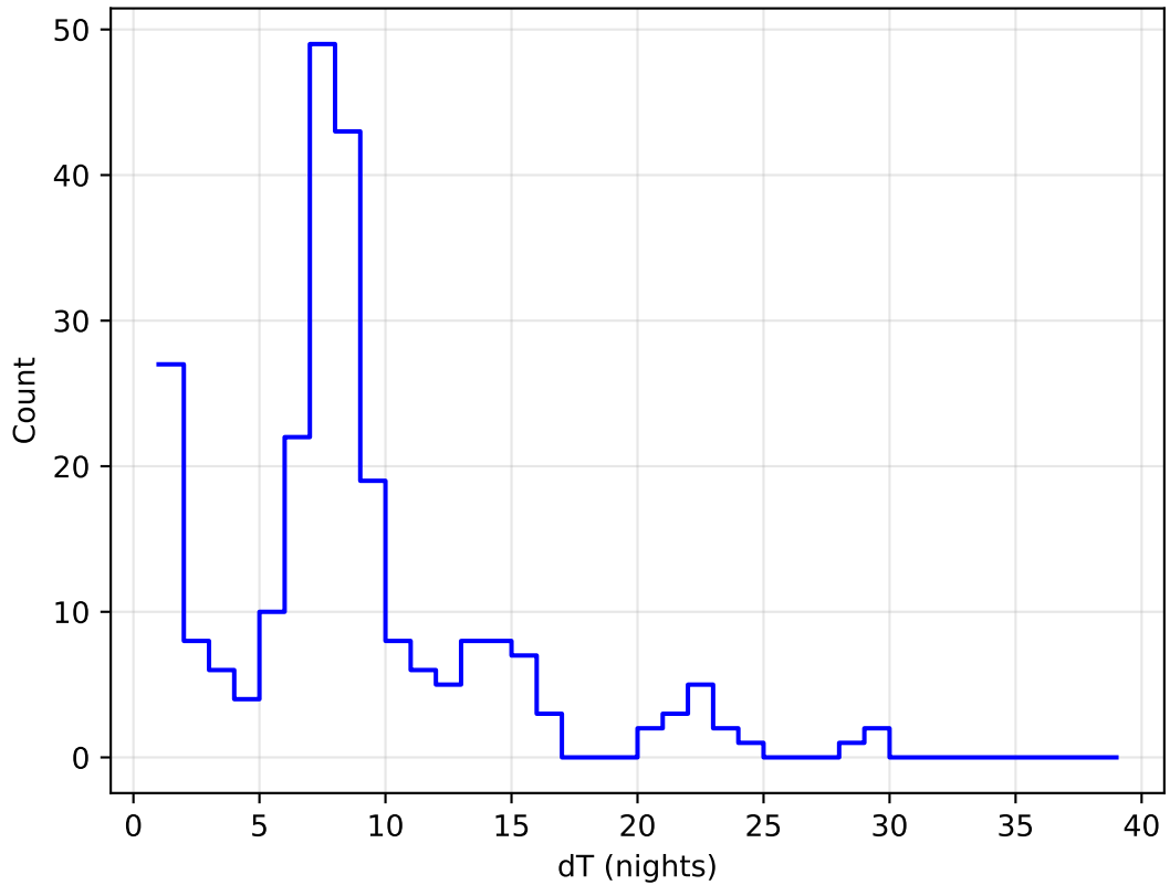
weather_cloudso36v3.4_10yrs all bands: DD:ECDFS Delta Nights Histogram
