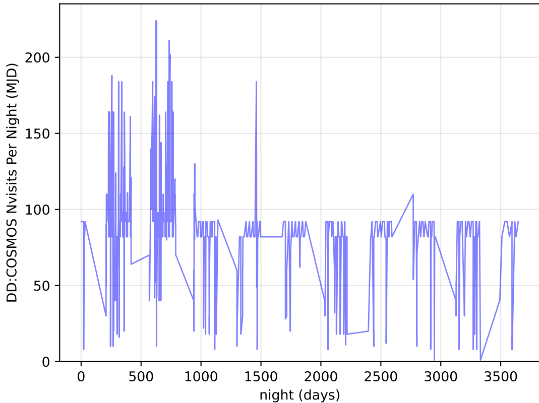
weather_cloudso36v3.4_10yrs all bands: DD:COSMOS Nvisits Per Night
