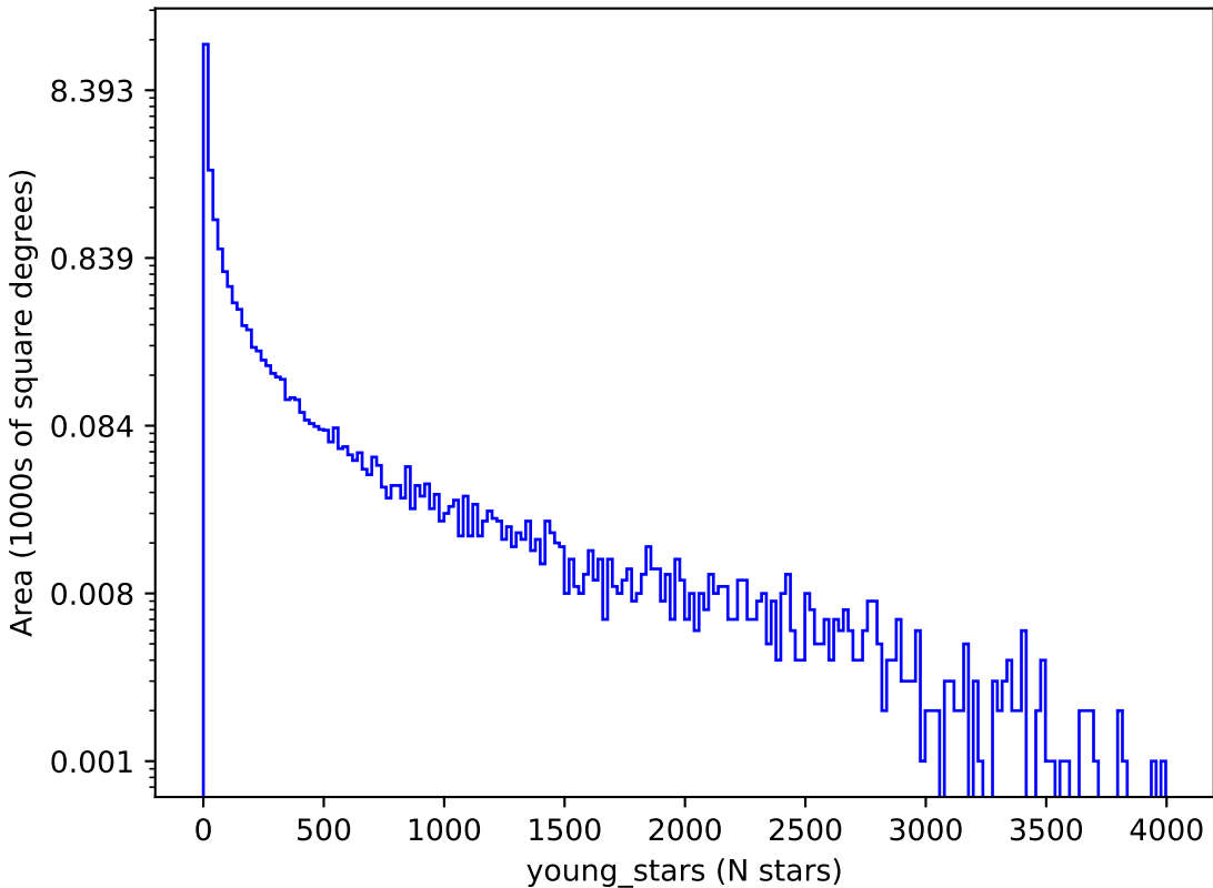
weather_cloudso35v3.4_10yrs : young_stars
