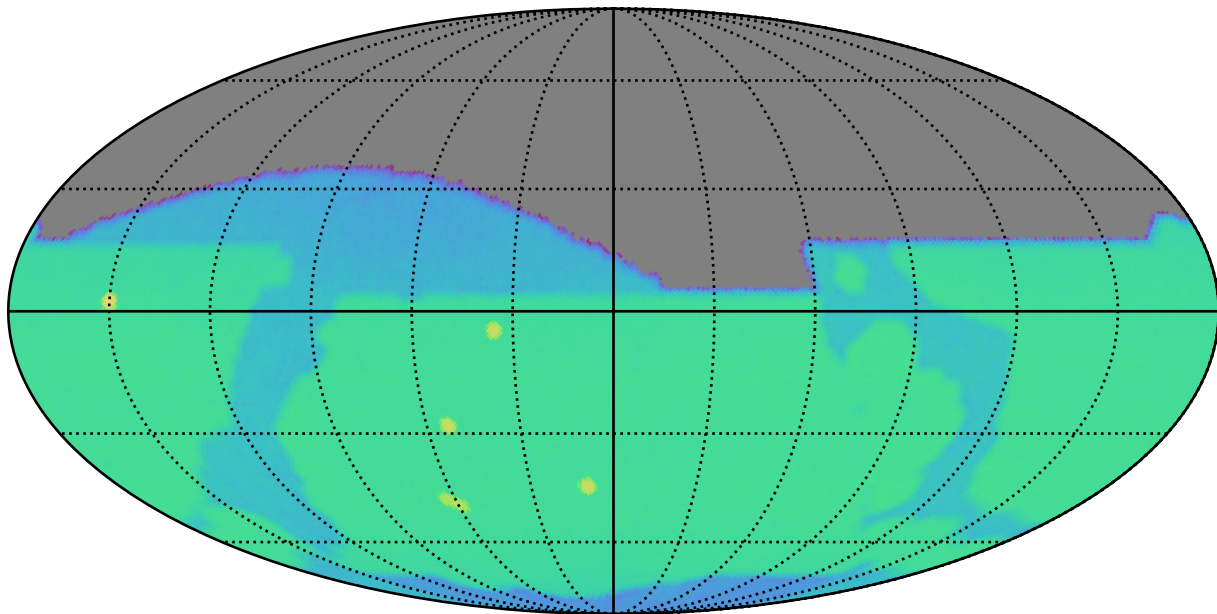
weather_cloudso35v3.4_10yrs i: SurfaceBrightLimit
