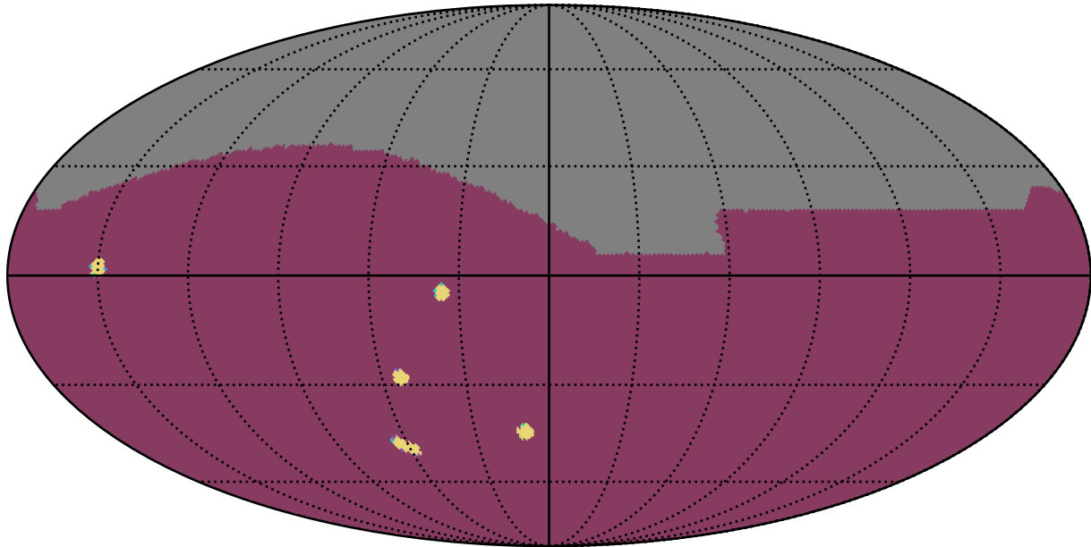
weather_cloudso35v3.4_10yrs : NumberOfQuickRevisits
