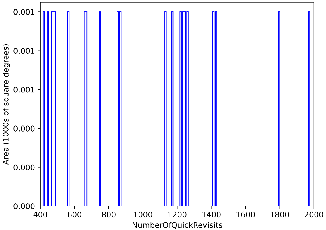
weather_cloudso35v3.4_10yrs : NumberOfQuickRevisits
