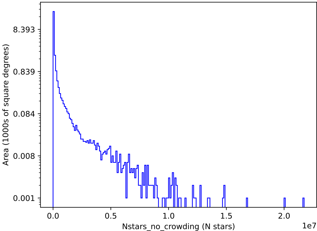
weather_cloudso35v3.4_10yrs r: Nstars_no_crowding
