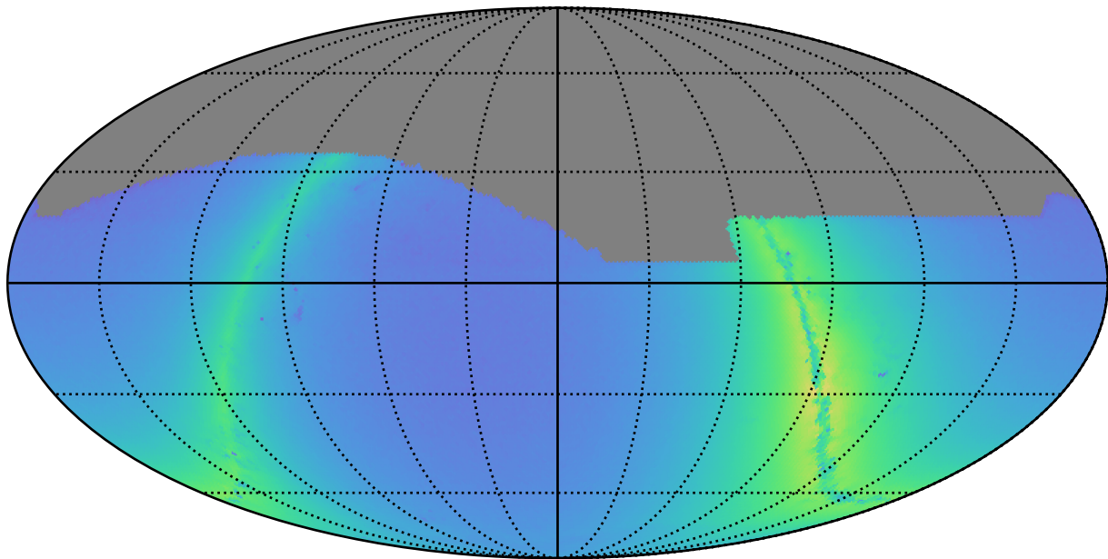
weather_cloudso35v3.4_10yrs i: Nstars_no_crowding
