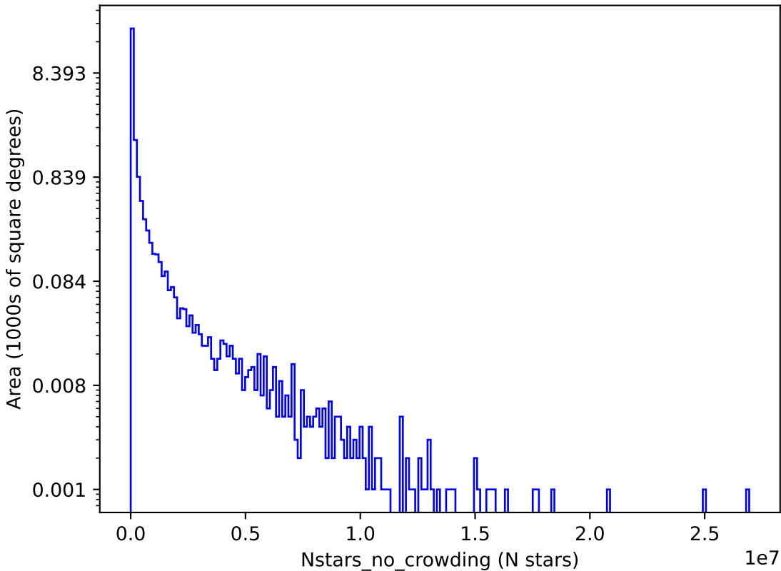
weather_cloudso35v3.4_10yrs i: Nstars_no_crowding
