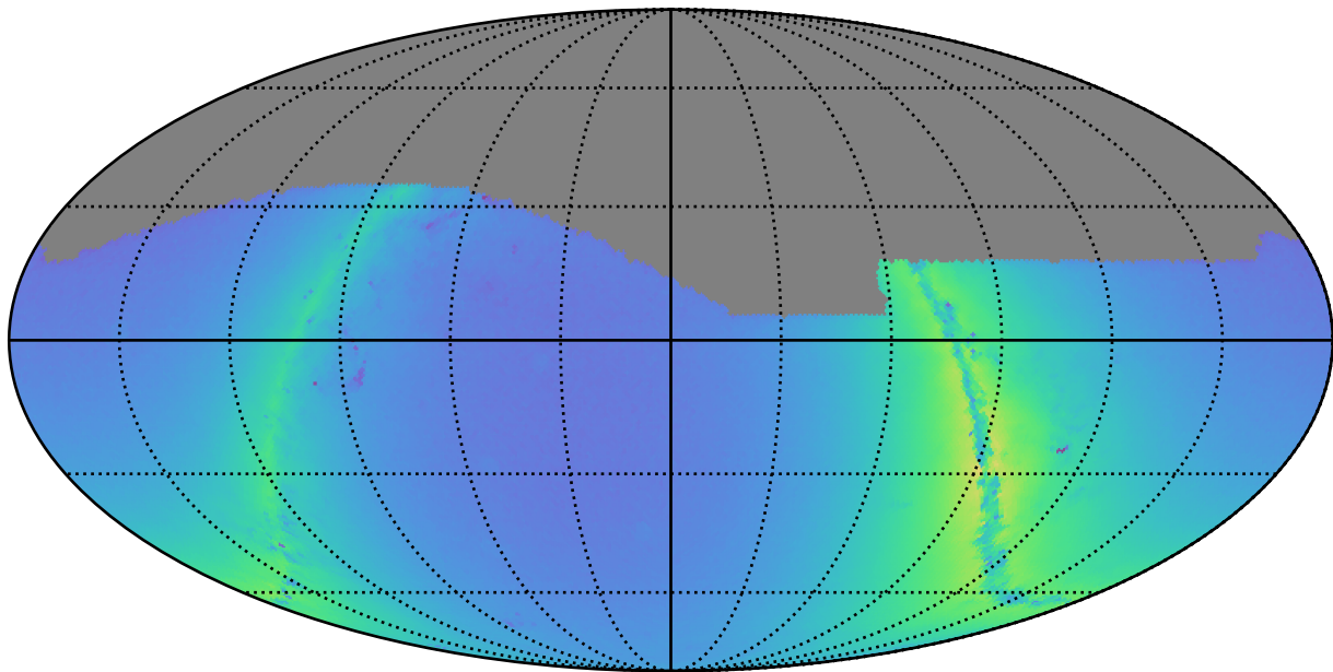
weather_cloudso35v3.4_10yrs g: Nstars_no_crowding
