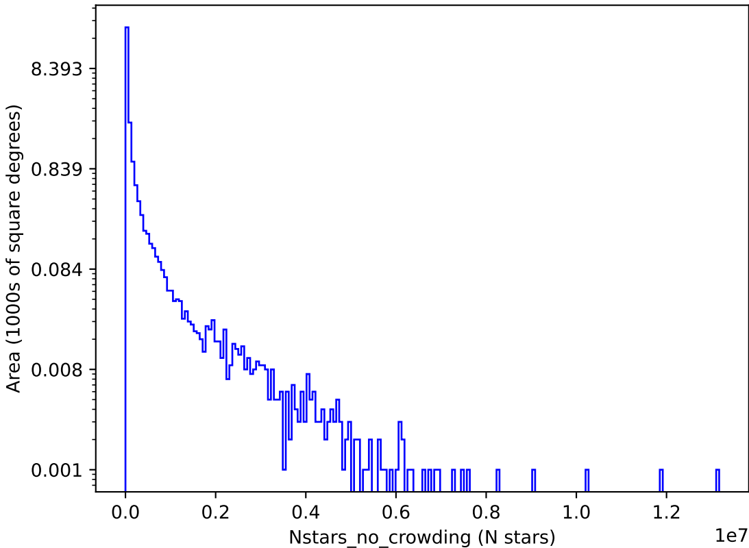
weather_cloudso35v3.4_10yrs g: Nstars_no_crowding
