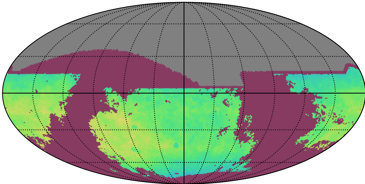
weather_cloudso35v3.4_10yrs i: NgalScale
