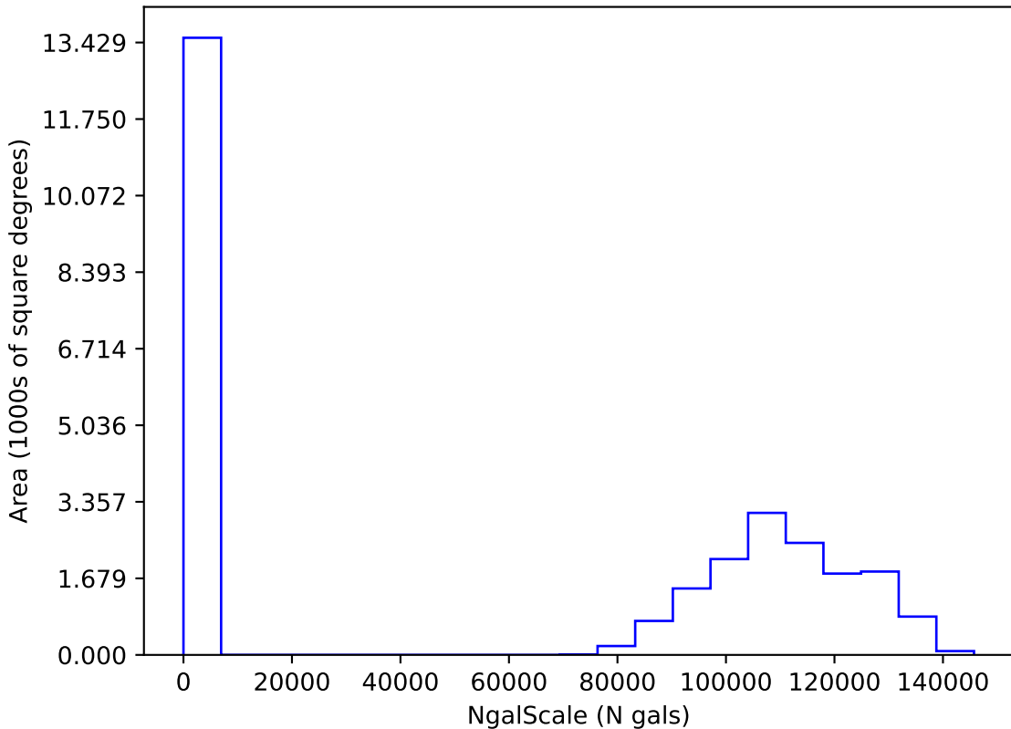
weather_cloudso35v3.4_10yrs i: NgalScale
