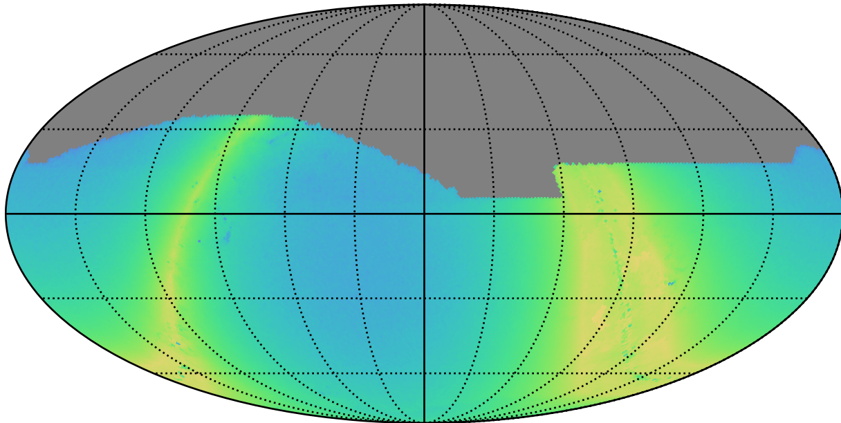
weather_cloudso35v3.4_10yrs i: N stars to Precision 0.20
