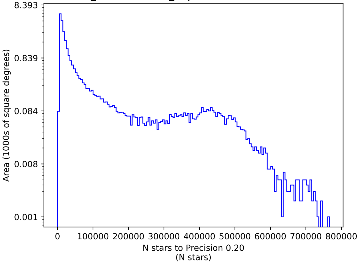
weather_cloudso35v3.4_10yrs i: N stars to Precision 0.20
